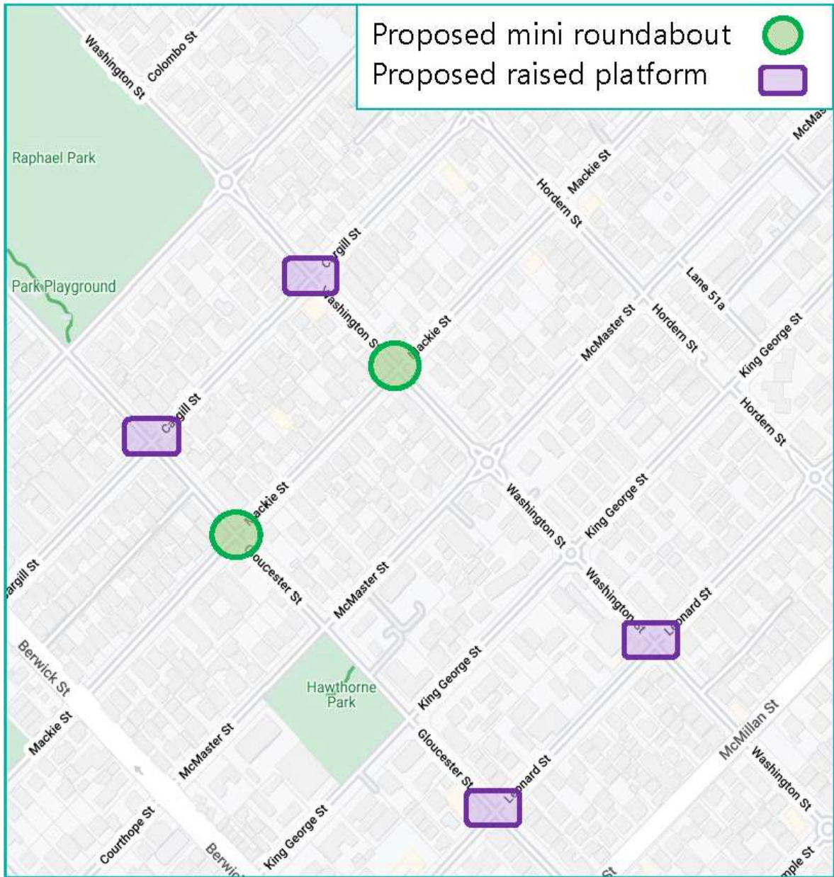
Mini roundabout example
